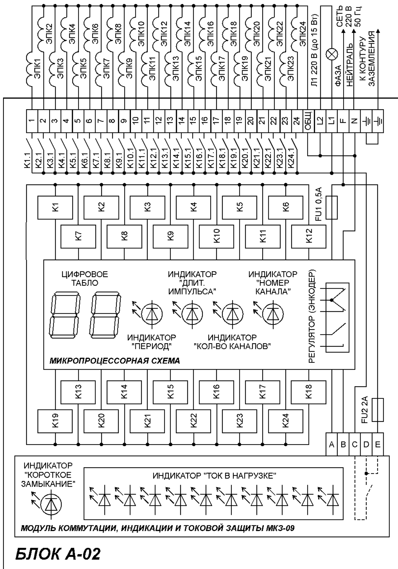
Рис. 2. Схема подключения и органы управления блока А-02.
